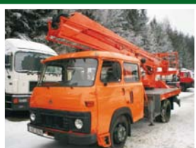
AVIA A 31 TL, MP 16 r.v. 1995 double kabina, po střední opravě
